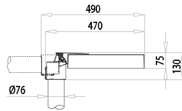
TP Ø76
