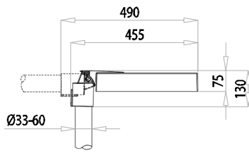
TP Ø60
