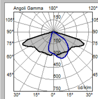
Ottica STU-M
