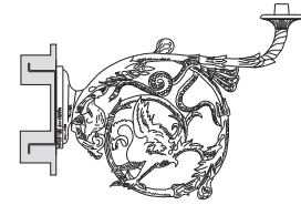
BR 10 Sporgenza / Projection mm 750 KG 34
