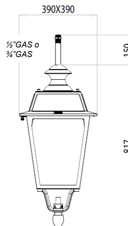
FIRENZE EVO S Installazione Sospesa 1/2" GAS o 3/4" GAS Attacco L=150mm
