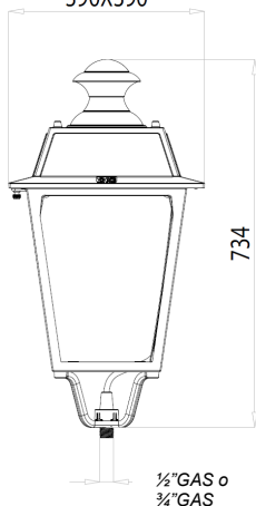
FIRENZE EVO Installazione portata 1/2" GAS o 3/4" GAS 390X390
