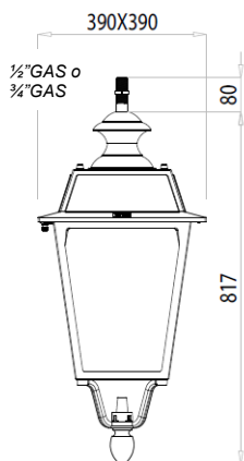
FIRENZE EVO S Installazione Sospesa 1/2" GAS o 3/4" GAS Attacco L=80mm
