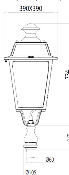
FIRENZE EVO Installazione portata per cima-palo ø60mm 390X390
